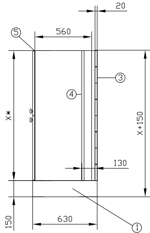
Схема установки корпусов
