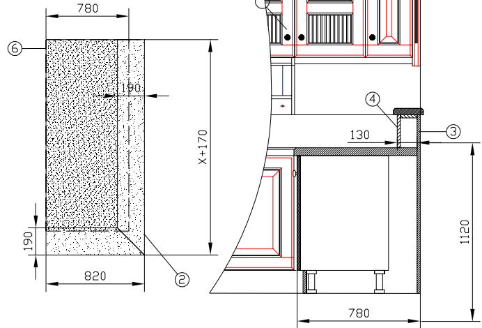
Схема установки столешниц
