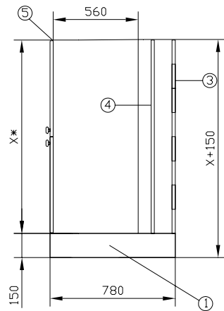
Схема установки корпусов
